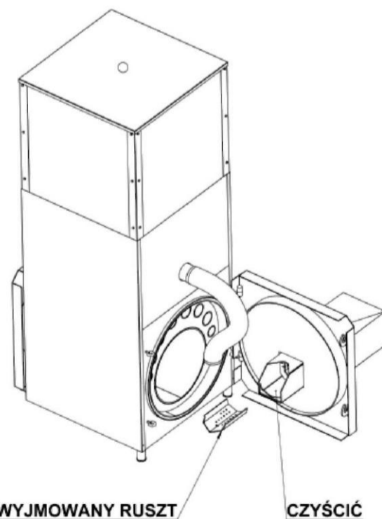
Рис. 08. Чистка форсунки
