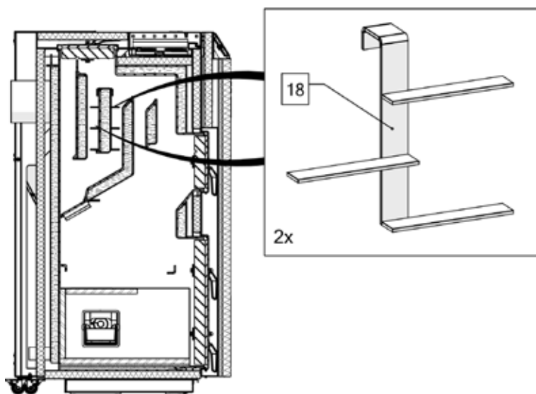
Rys: Rysunek 4. Zestaw zawirowywaczy oraz ich umiejscowienie w kotle Twin Bio Luxury Compact typ NE 16 – 24
